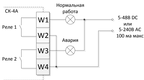
Рисунок 4.2 – Выходные цепи
